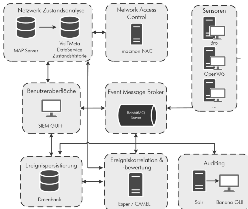
Abb. 1: CLEARER-Architektur in der Gesamtübersicht
