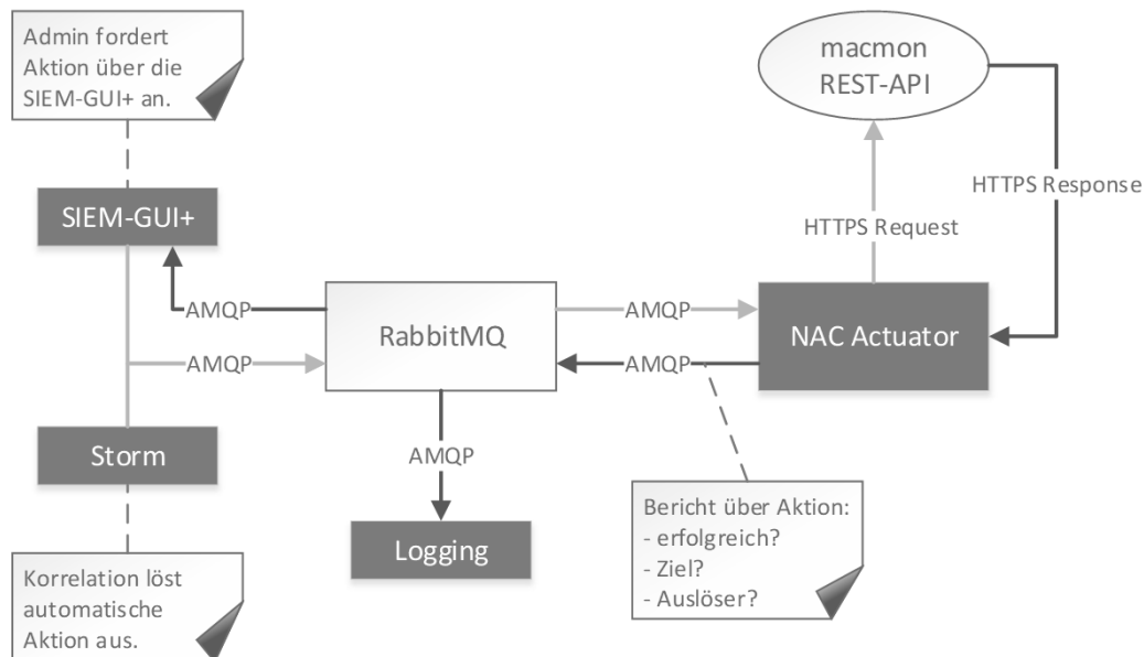
Abb. 4: NAC-Schnittstelle von CLEARER über REST-API
